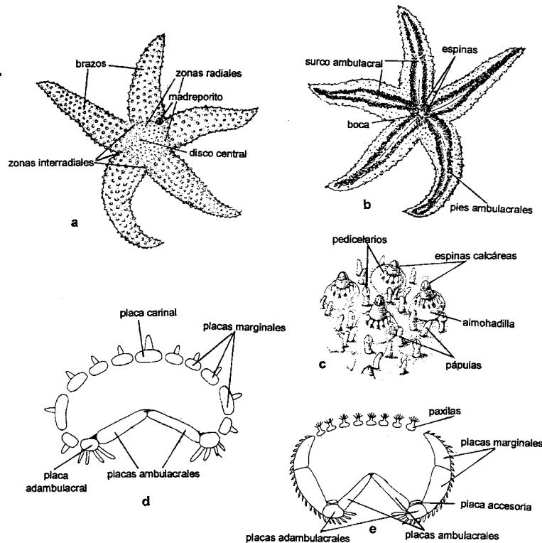
Asteroideos: a) aspecto general de la cara aboral; b) aspecto general de la cara oral; c) detalle de la superficie aboral; d) sección de un brazo de Marthasterias sp. ; e) sección de un brazo de Astropecten sp.
