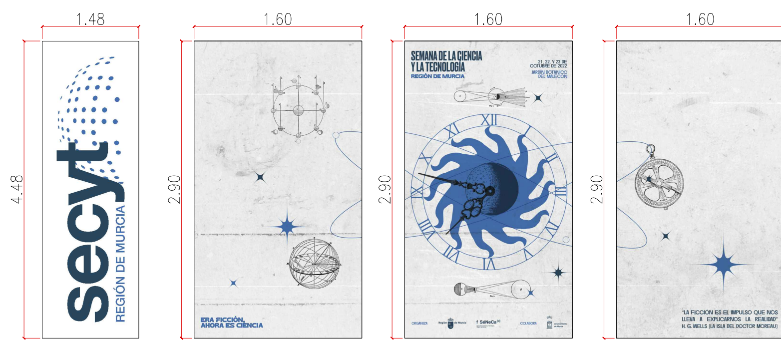
1a TORRE ENTRADA. PARTE SUPERIOR 2 UNIDADES VINOLO DE CORTE SOBRE ALUCOBOND BLANCO
