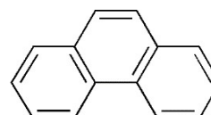
fenantreno
